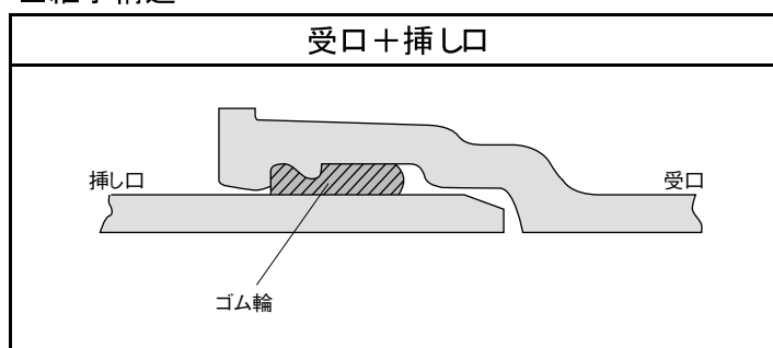
■継手構造
